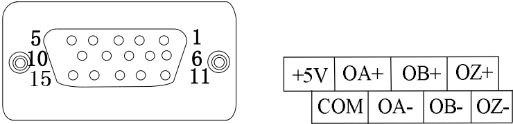
附录 B：图 7 680-PGS 端子图
