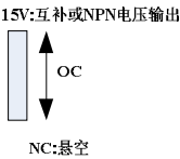
附录 C：图 3 680-PGC 跳线开关图
