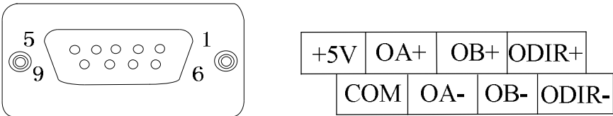
附录 B：图 5 680-PGR 端子图
