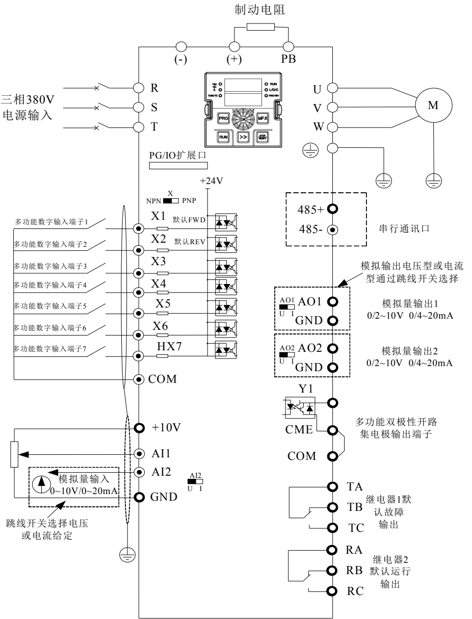
图 3-2. 三相 380V 0.75~ 30kW（4T:380V）及单相 220V（2S）5.5kW 以下(输入接 R T)变频器接线图
