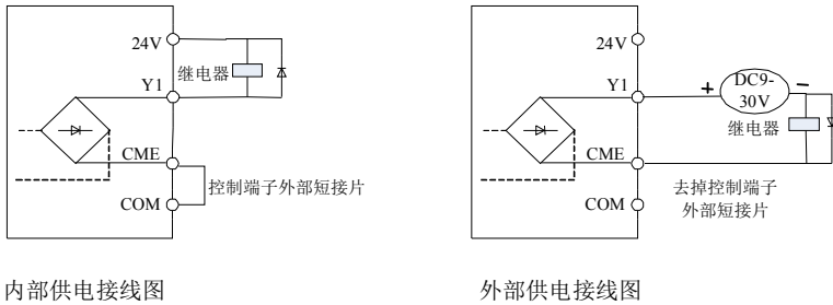
图 3-12. 数字输出端子Y1 接线示意图
