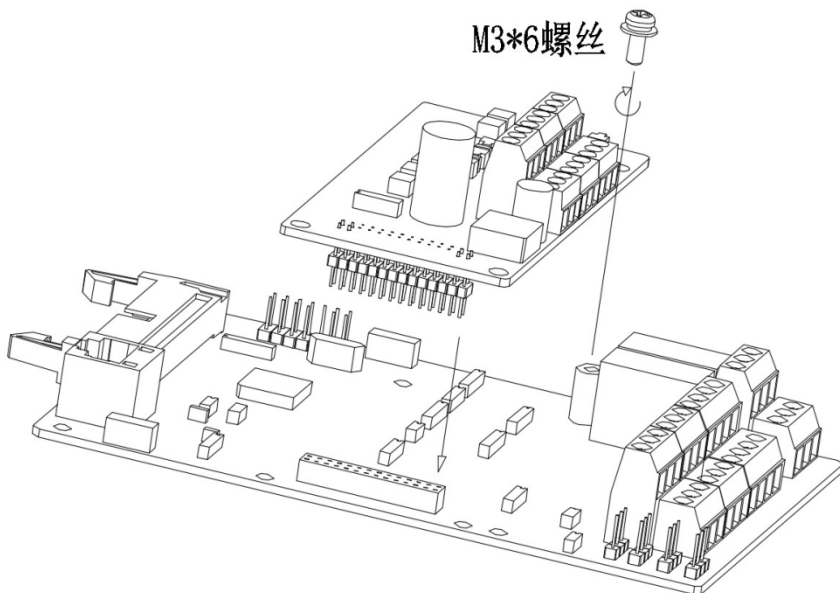
附录 C：图 1 高性能闭环驱动器扩展卡安装方式
